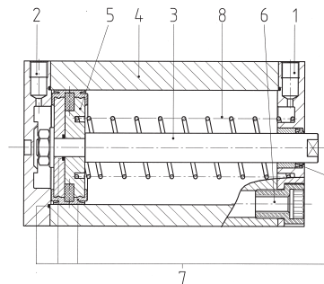
tipo CUS...-FA; CUS...-FP; type CUS...-MA; CUS...-MP
