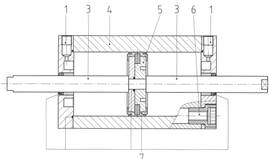
tipo CUSP...-F; CUSP...-M; CUDP...-F; type CUDP...-M; CUSP...-M4; CUDP...-M4
