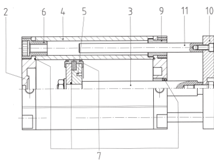
tipo CUD...-A; CUDP...-A type
