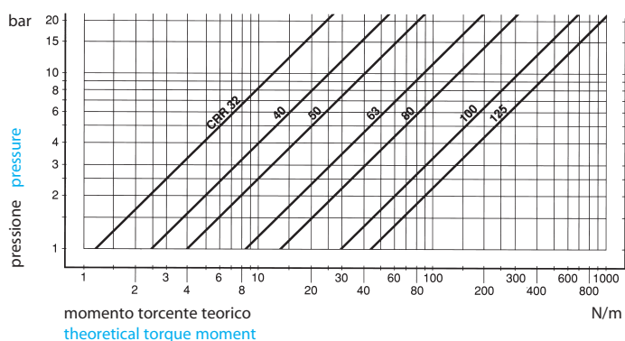
Fig. 4 Diagramma momento torcente - pressione (1 Nm \approx 0,1 kpm) Diagram torque moment - pressure (1 Nm \approx 0,1 kpm)
